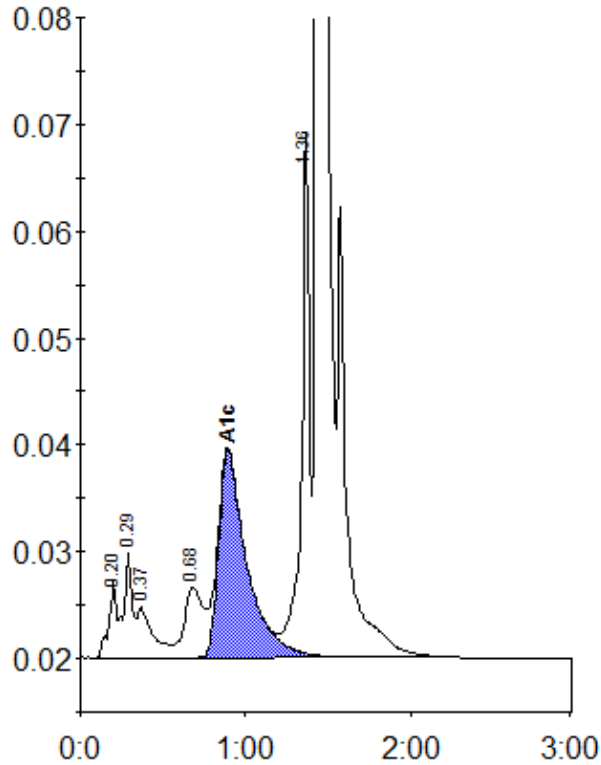
Peak table - ID: 10568179
